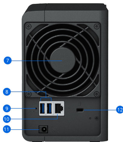
DS223 (vzadu)
